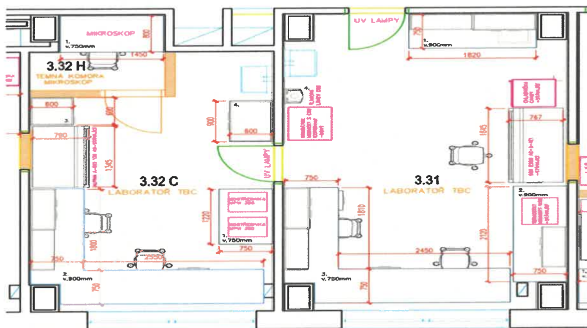
3.31 LABORATOŘ TBC, 3.32C LABORATOŘ TBC A 3.32H TEMNÁ KOMORA, MIKROSKOP — půdorys
