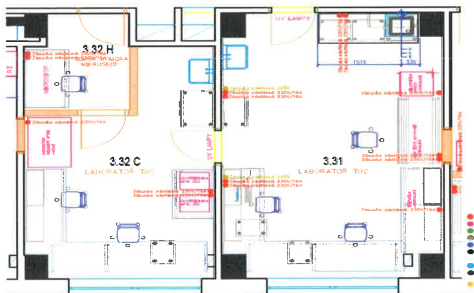
3.31 LABORATOŘ TBC, 3.32C LABORATOŘ TBC A 3.32H TEMNÁ KOMORA, MIKROSKOP – napojovací místa
