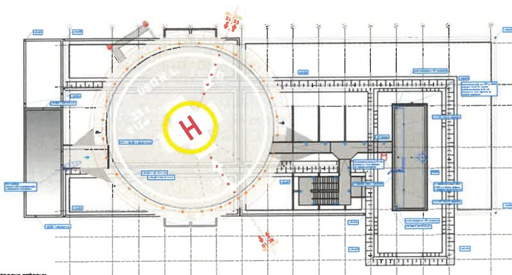
PODORYS STŘECHY
